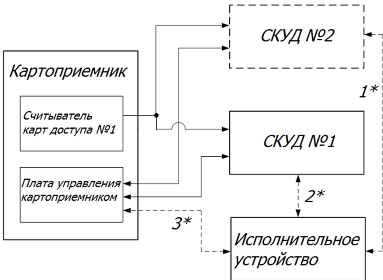
Рис. 19. Структурная схема №2
